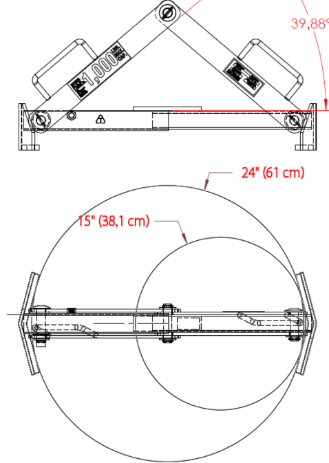
Modell 92-30 und 92-30SS
