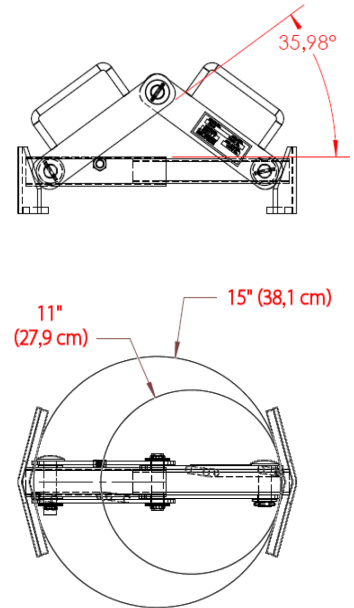
Modell 92-5 und 92-5M
