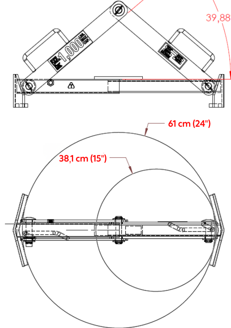
Modelos 92-30 y 92-30SS
