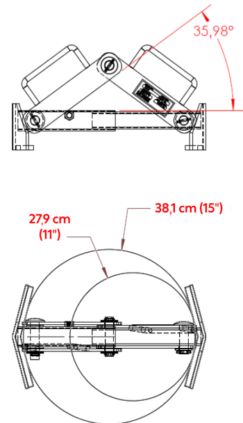
Modelos 92-5 y 92-5M
