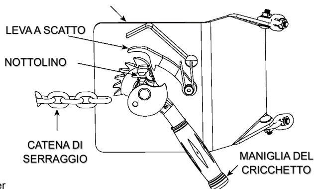
PIASTRA DI CERNIERA A CRICCHETTO
