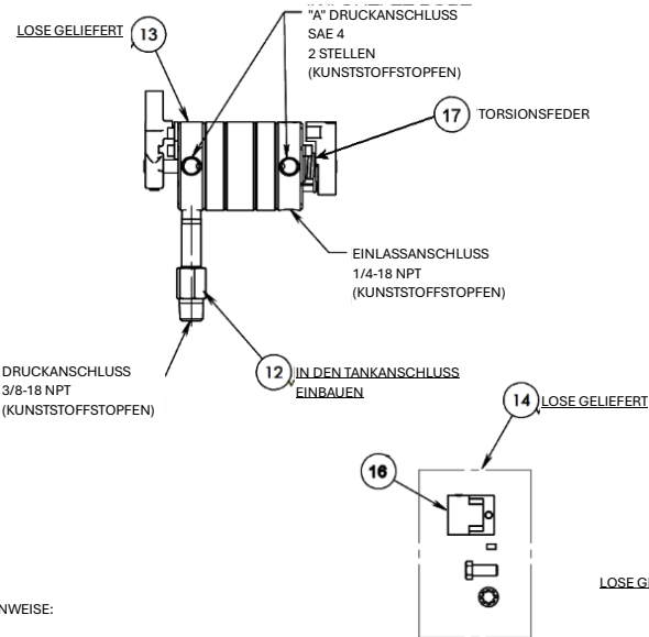
SCHEMATISCHER AUFBAU
