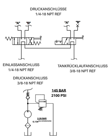
SCHEMATISCHER AUFBAU
