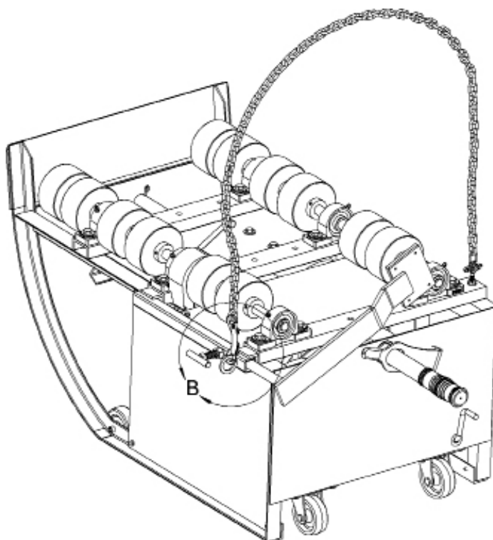
Rodillo para bidones portátil Morse Se muestra con la opción POLY-201 instalada de fábrica
